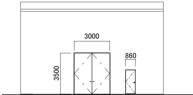
西側立面図 1/200
